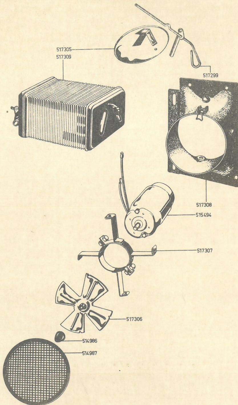
Gruppe 35-Klimaanlage - Einzelteile Group 35-Heater-Assy.(Component Parts) Bildtafel Nr. 113 Illustrated Plate No. 113
