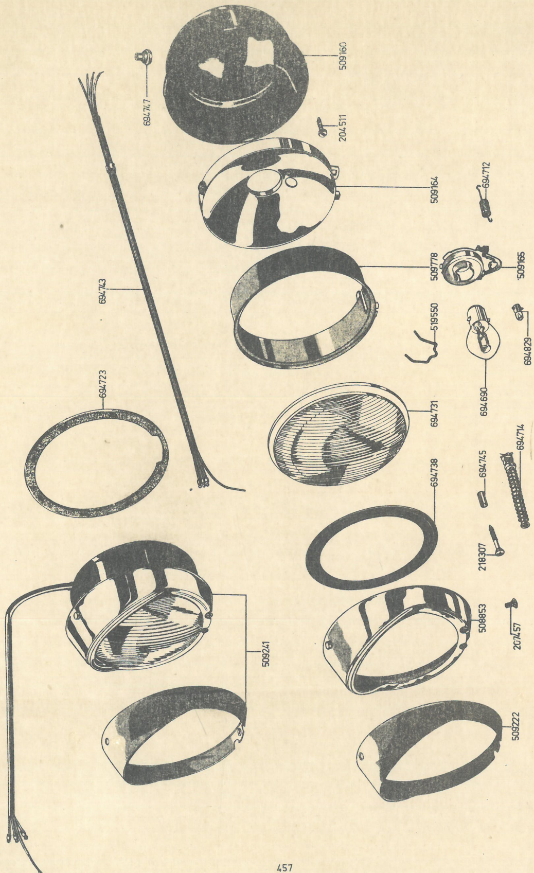
Gruppe 13B-Scheinwerfer symmetrisch Group 13B-Head Lamps Symmetrical Bildtafel Nr.90 Illustrated Plate No.90
