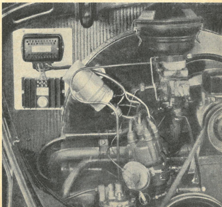
Fig. 2. Det kompakte anlæg med 3 helt indkapslede enheder monteret i en VW.
