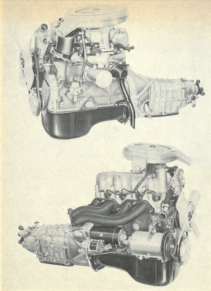
Motoren i FIAT 1500 udvikler 80 HK (SAE), med et volumenindhold på 1481 ccm. De elegant svungne udblæsningsrør letter i høj grad gasafgangen.
