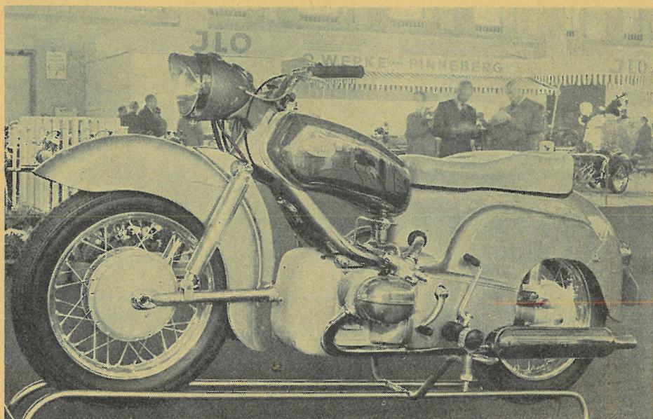
Zündapp's ny 250 ccm model med boksermotor. Stelkonstruktionen er meget særpræget, og motoren er monteret i fjedrende trepunkt-ophængning. Begge hjul er affjedret ved hjælp af svinggaffler. Det ene gaffelben i baggaflen tjener tillige som kardantunnel.
