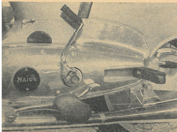
Som vist på nedenstående, forsvinder den bageste fodhviler ind i motorblokken på Maico Taifun. Også på denne side findes et gummidæksel, bag hvilket den anden karburators dyser er tilgængelige. Over dækslet ses tipperarmen.
