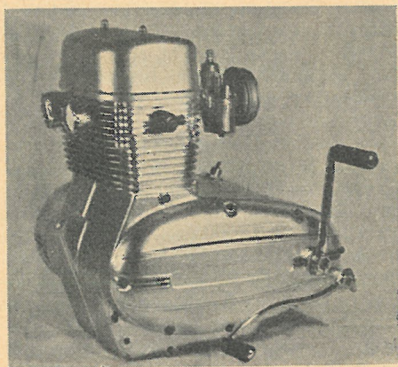
Den i teksten omtalte to-cylindrede Opti motor med overliggende knastaksel. Denne motor er særpræget, fordi såvel krumtapaksel som krumtaplejer er udelelige.
