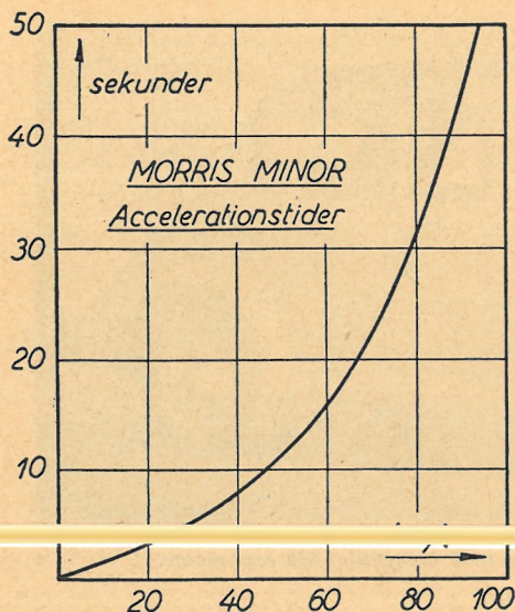
Accelerationkurven for Morris Minor viser, at det er en levende, lille vogn.
