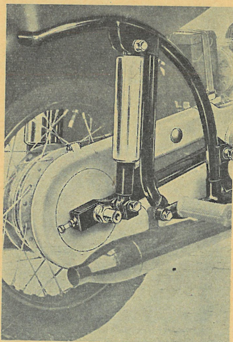
Baghjulsaffjedringen på den »konfektionssamlede« Thornax. Som det ses, er såvel lyddæmpere som de bageste fodhvilere i fast forbindelse med stelkonstruktionen.
