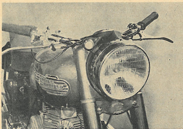
Forpartiet af Royal Enfield »Meteor«. Som det ses er forgaflen, speedometeret, lygten og kontakterne bygget sammen i en konsol, der tillige bærer to parkeringstygter. Bemærk de to kabler fra bremsehåndtaget.
