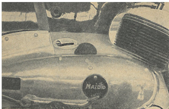
Friløbshåndtaget ses her på Maico Taifun. Foran og under håndtaget sidder et gummi-dæksel, der giver adgang til karburatorernes dyser. På det sted, hvor lænderørskablerne forsvinder ind i stellet, presses også indsugningsluften ind.
