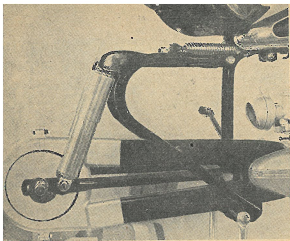
Jurisch fjederelementer og lukket kædekasse. Den del af kædekassen, der ligger omkring det medens kædelunetterne er udførte i hårdvulkaniseret, syntetisk gummi.
