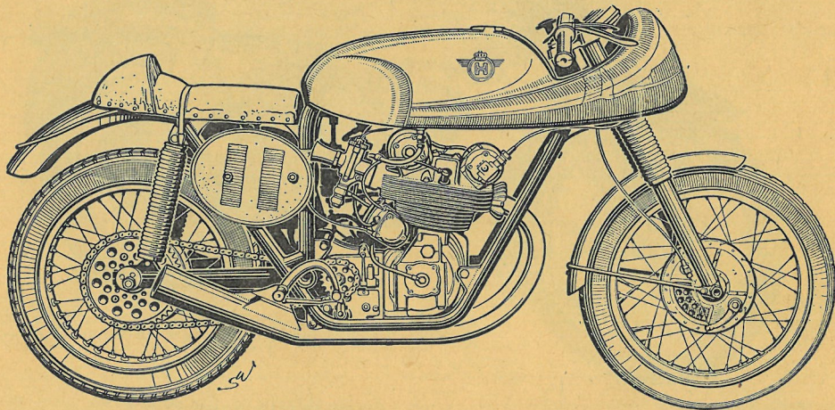
En stregtegning af Horex raceren med to-cylindret motor og to overliggende knastakslers. Bemærk stelkonstruktionen, der er udført af forholdsvis stordimensionerede, tyndvæggede rør. Benzintanken er fremstillet af aluminium og er banket op i hånden.
