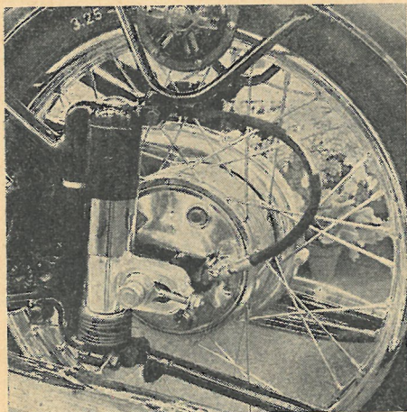
Den hydrauliske baghjulsbremse på TWN modellerne. Der er to fordele ved dette bremse-system: for det første er bremsevirkningen blød på den første del af pedalvandringen, medens blokering først finder sted ved hård aktivering. For det andet giver den hydrauliske bremse lettere tilslutningsmulighed for en sidevognsbremse.
